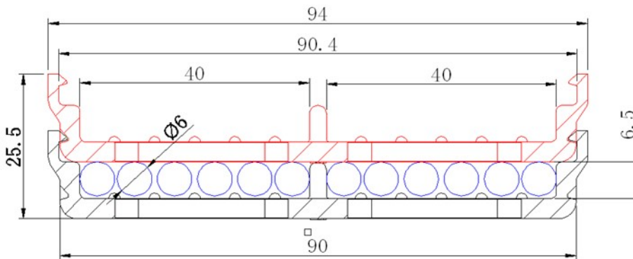
φ6x12固线器组装示意图
