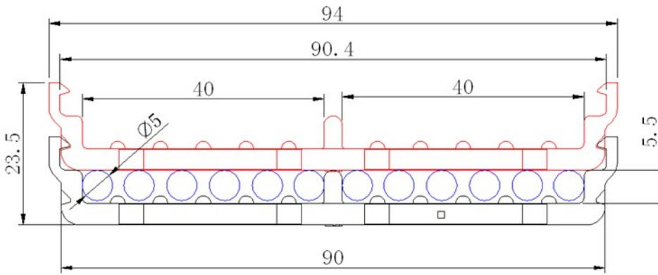
φ5x12固线器组装示意图
